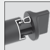
Molette easyclean – positionnez-le correctement (picot à l'intérieur de l'évidement)
