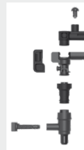
Pièces détachées de la buse à vapeur
